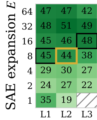
SleepFM
